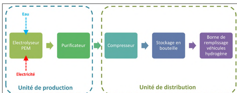
Process de l'unité de production et de distribution d'hydrogène
